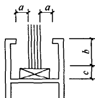
图 5.3.2-1 单片玻璃、夹层玻璃、真空玻璃最小安装尺寸
