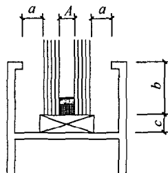
图 5.3.2-2 中空玻璃最小安装尺寸
