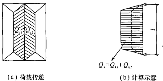
图 B. 0.1-3 双扇门窗荷载传递
