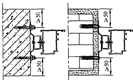
图 7.3.1-2 固定片与墙体位置
