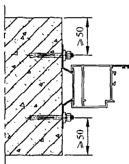
图 7.3.2-1 卡槽连接方式
