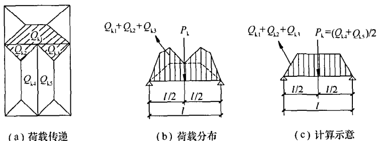
图 B. 0. 1-4 带上亮双扇门窗荷载传递
