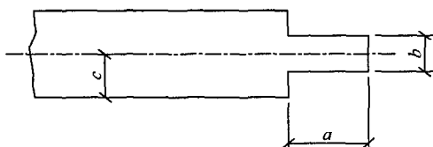
图 6.2.2-3 构件的榫头加工
