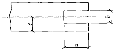
图 6.2.2-2 构件的豁口加工
