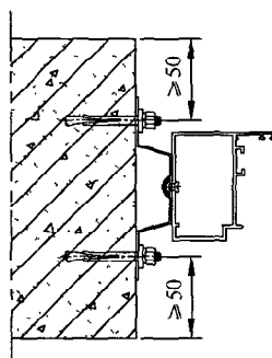
图 7.3.2-2 自攻螺钉连接方式
