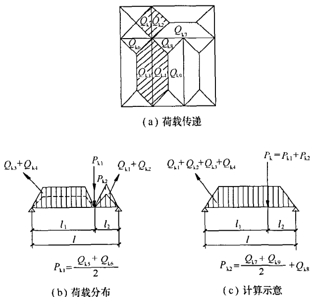
图 B. 0. 1-5 带上亮多扇门窗荷载传递
