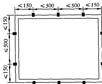
图 7.3.1-1 固定片安装位置
