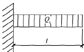
图 B.0.2-3 悬臂梁矩形分布荷载
