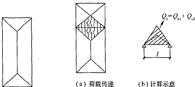
图 B. 0.1-1 单扇门 窗荷载传递
